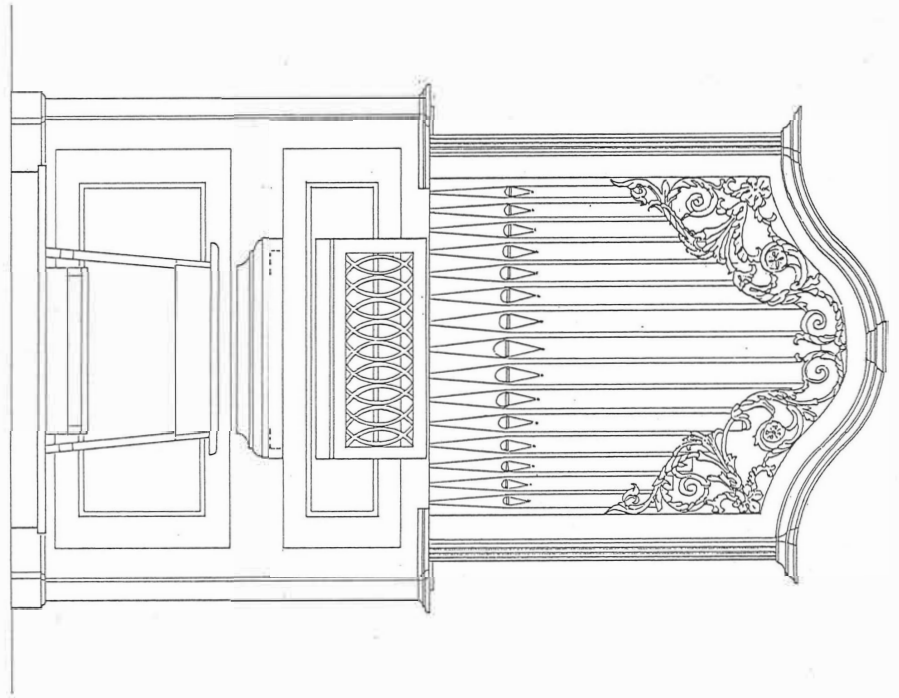
ELEVATION FRONTALE
